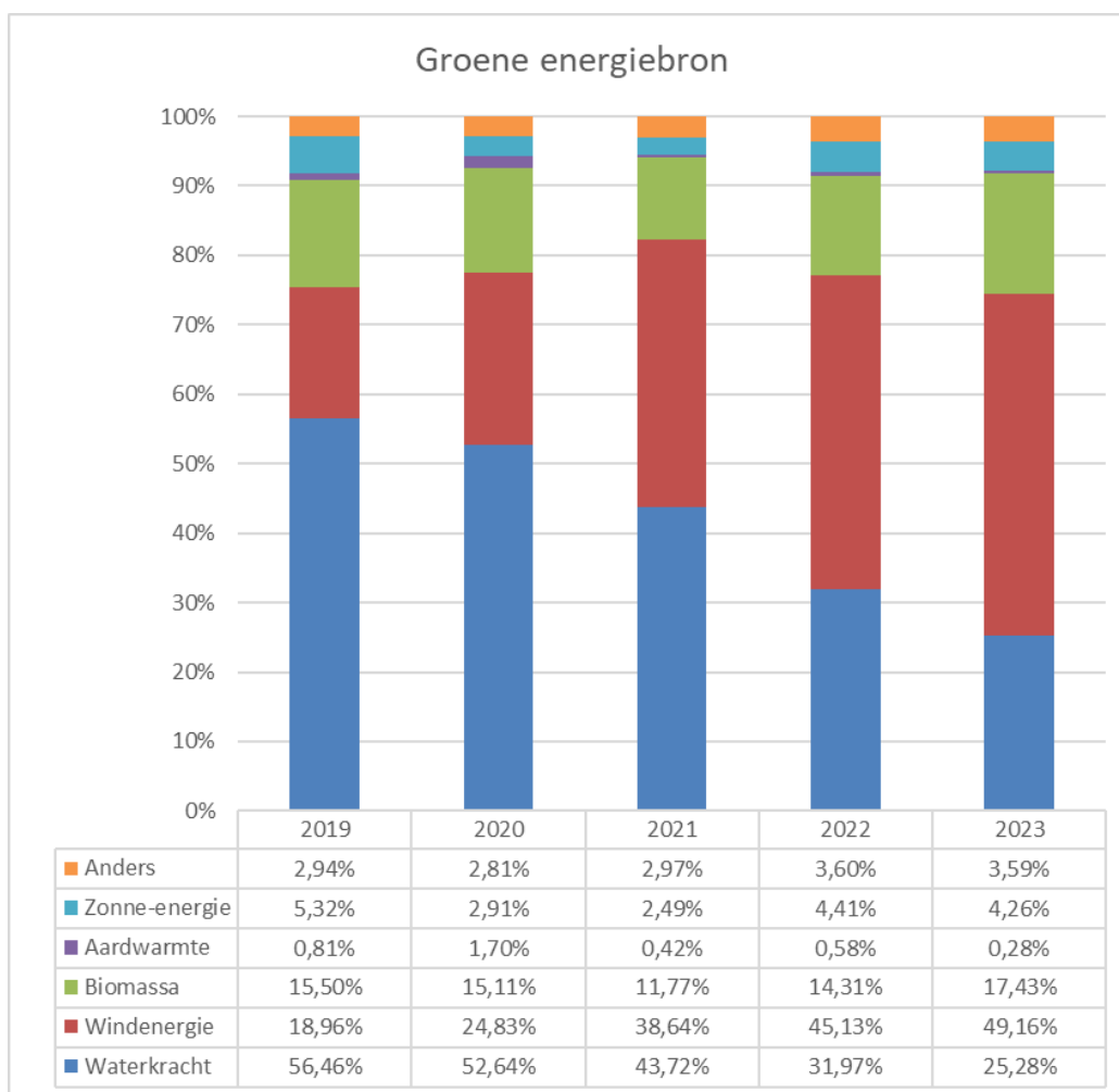
Figuur 7: Evolutie van de energiebronnen van de geleverde elektriciteit
